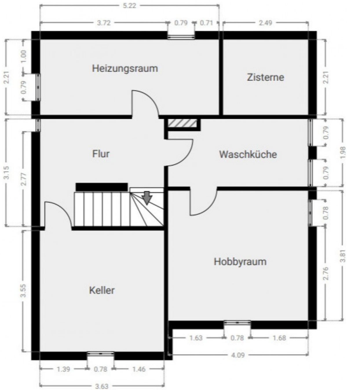
Grundriss Keller
