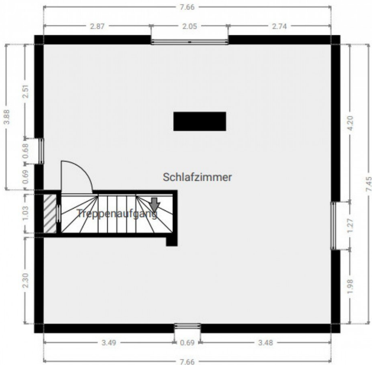
Grundriss Dachgeschoss
