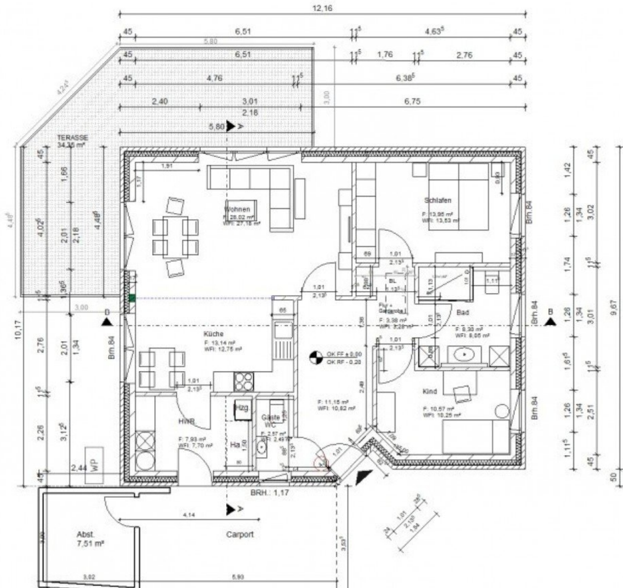
Grundriss Erdgeschoss
